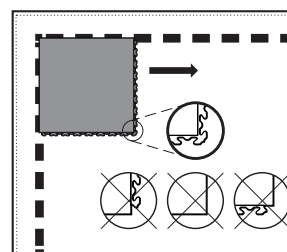
Obr. č. 3 Směr kladení dlaždic INVISIBLE, BUSINESS
